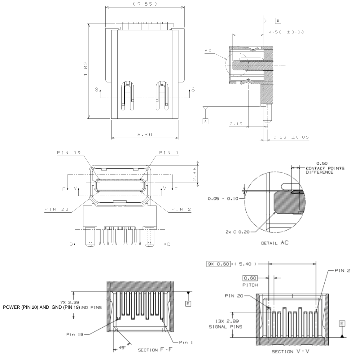
Figure 4-41: Mini DisplayPort Connector Dimensions - 1
