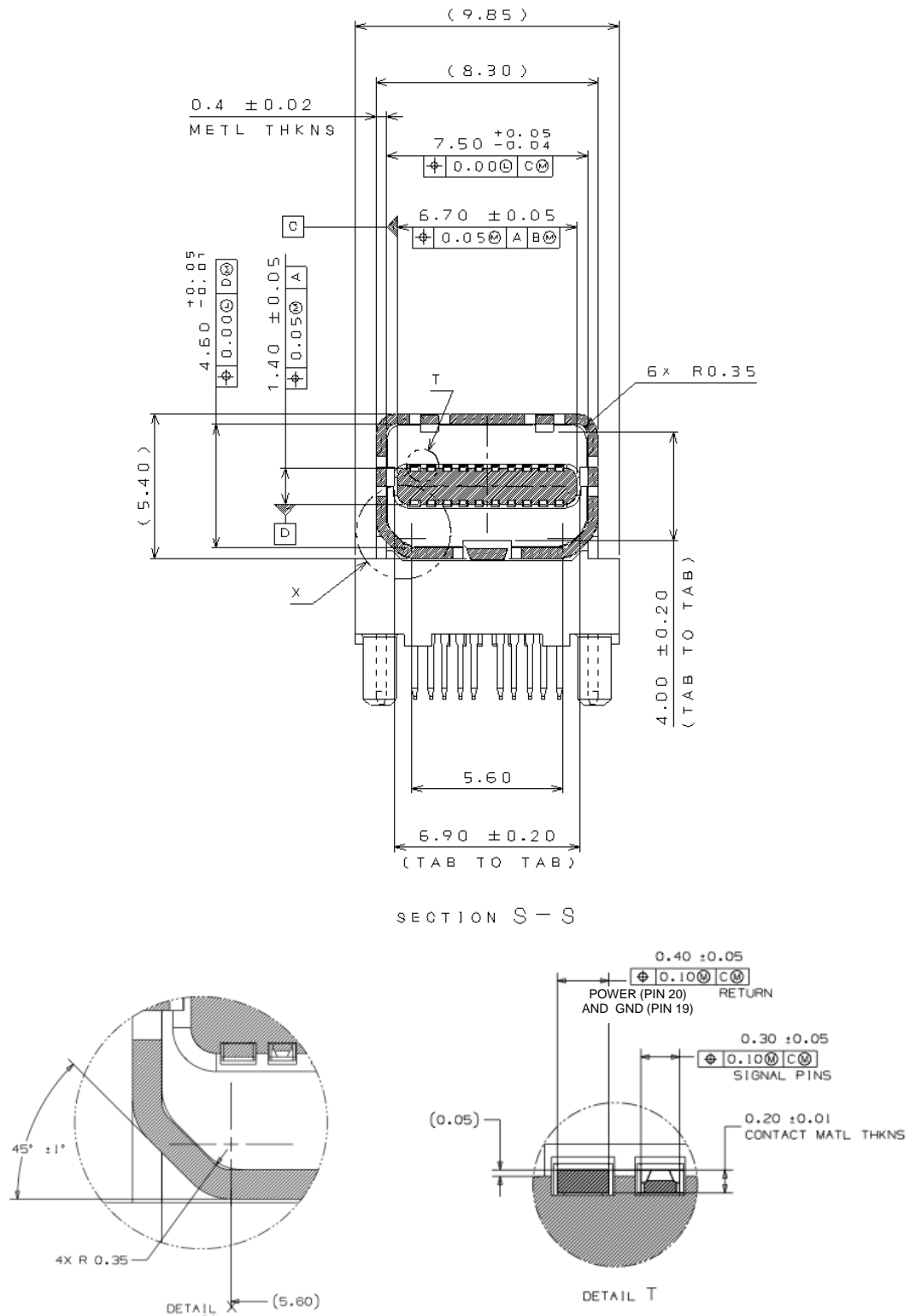
Figure 4-42: Mini DisplayPort Connector Dimensions – 2
